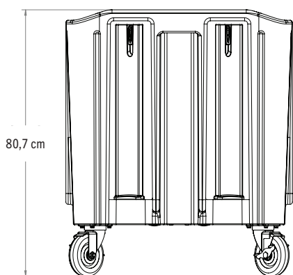
Modello: ADCSC12PKG con 12 torri
